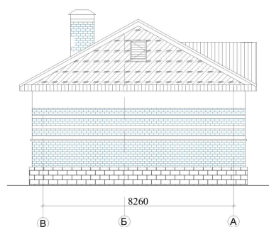
Вид справа
