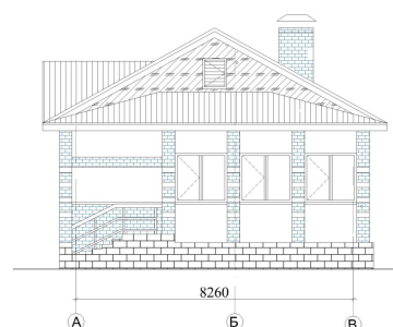
Вид справа
