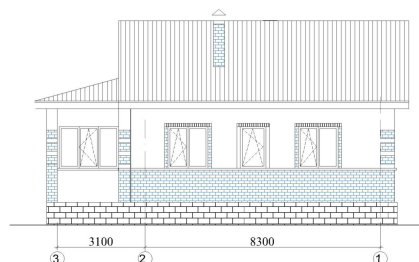
Вид сзади
