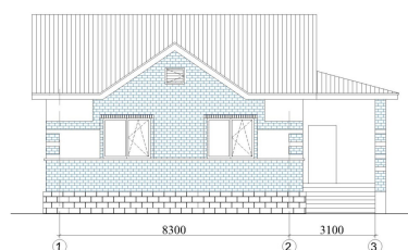
Главный фасад
